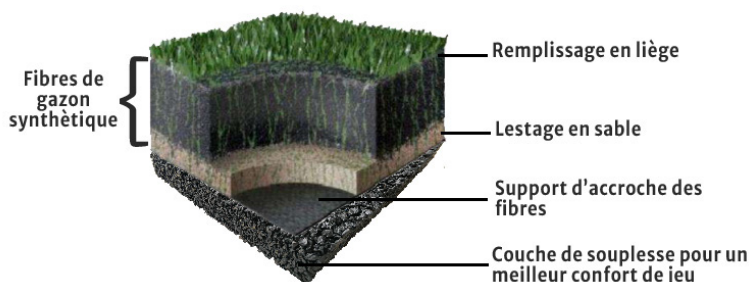
Schéma de la pose du gazon synthétique
