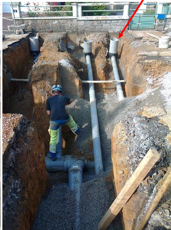
Boîte de branchement
